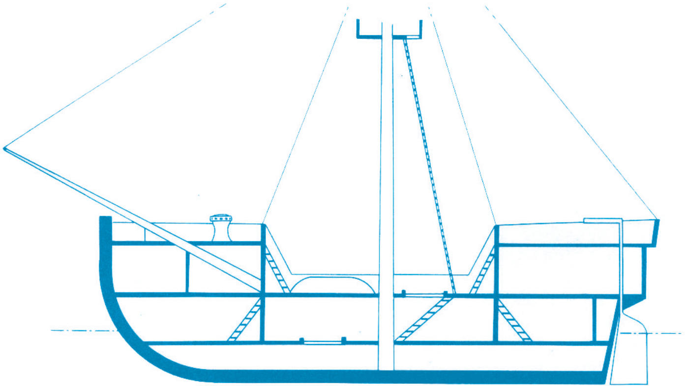
Sea Ghost longitudinal section
